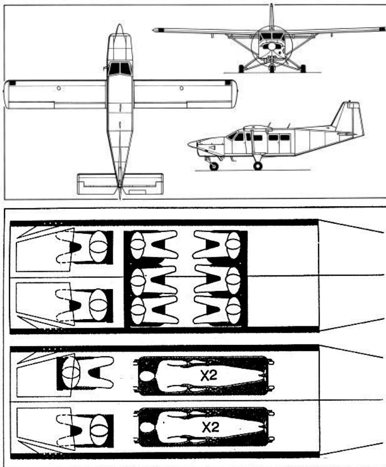
Esquemas del Gavilán G-358. Perfil de tres vistas y disposición de la cabina.
